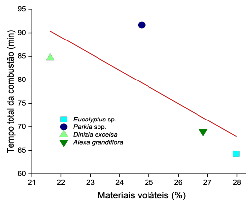
Figura 2: Correlação entre materiais voláteis e tempo de combustão.
